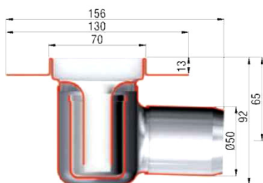
Standarta 92 mm kanāls ar atloku
