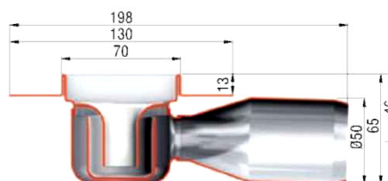
Pazemināts 65 mm kanāls ar atloku
